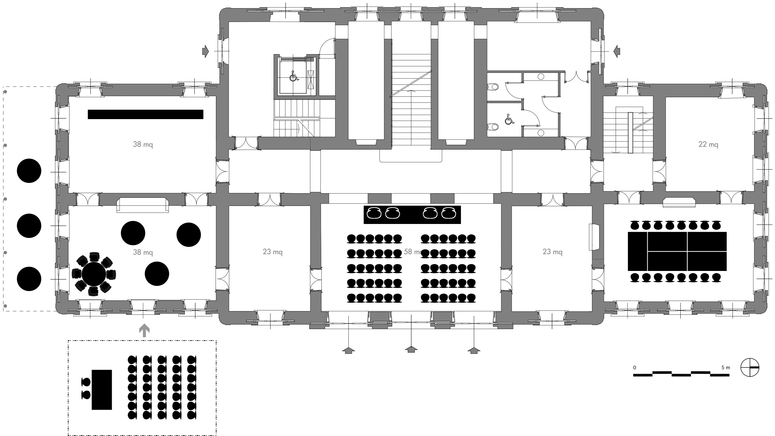
PIANTA PIANO TERRA: FUNZIONALE SCALA 1/100
